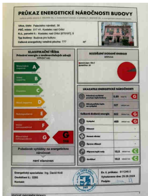
Obrázek 41 - Průkaz energetické náročnosti budovy Rabštejna
