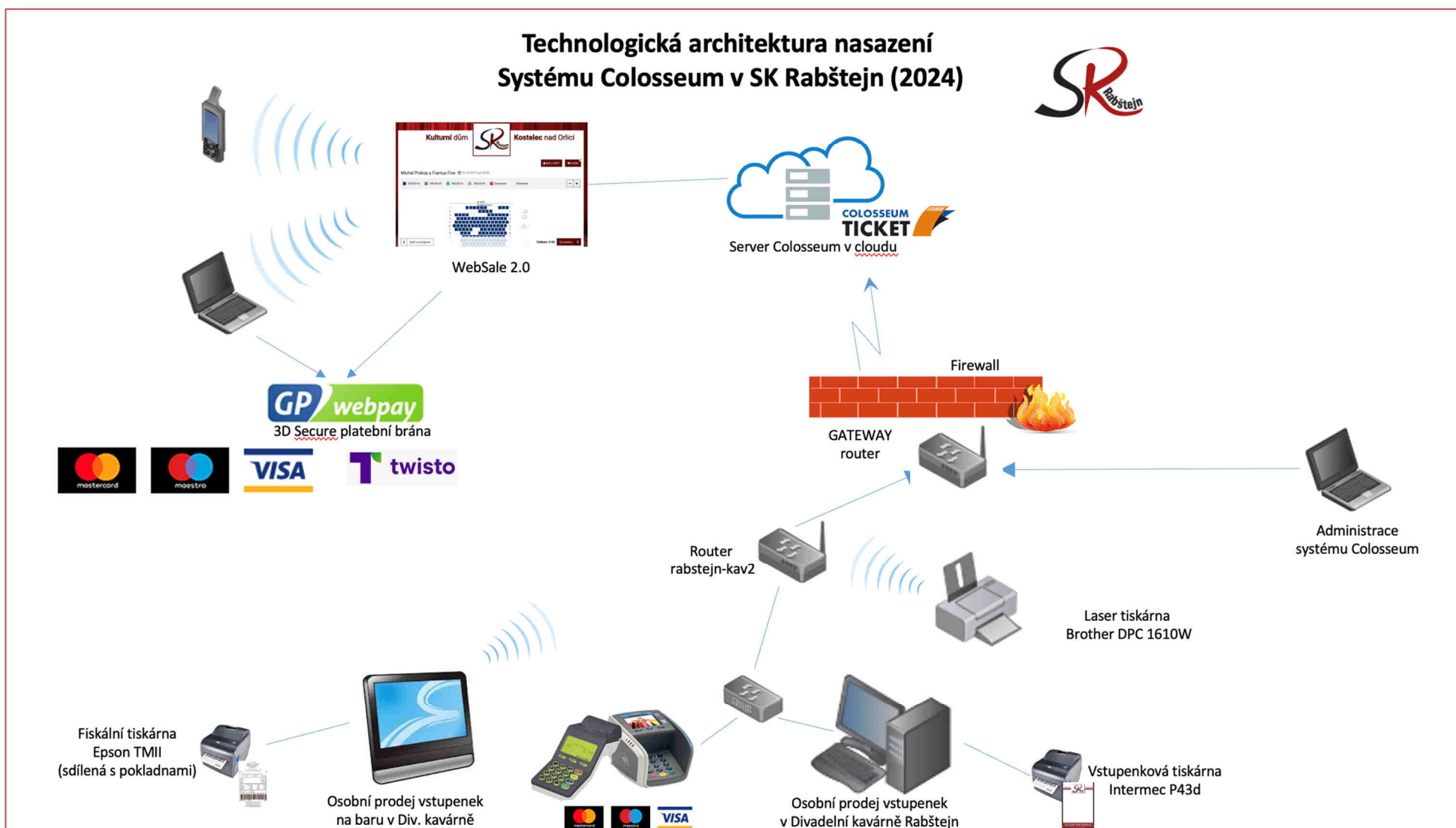
Obrázek 40 - Technologická architektura implementace Colosseum v roce 2024
