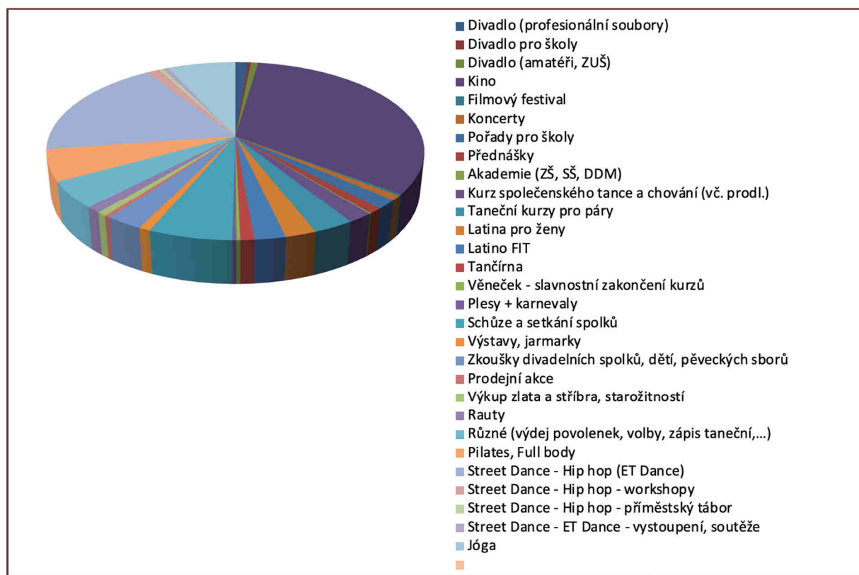
Obrázek 1 - Graf akcí
